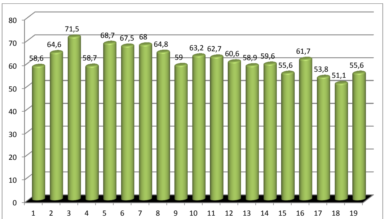
21 pav. Ekvivalentinio triukšmo pasiskirstymas matavimo vietose dienos metu (6-18 val.). Ribinis dydis 65 dBA.
