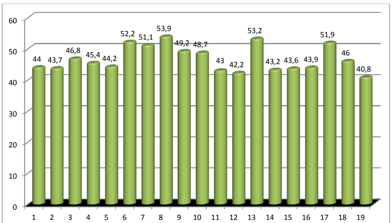
25 pav. Ekvivalentinio triukšmo pasiskirstymas matavimo vietose nakties metu (22-6 val.). Ribinis dydis 55 dBA.
