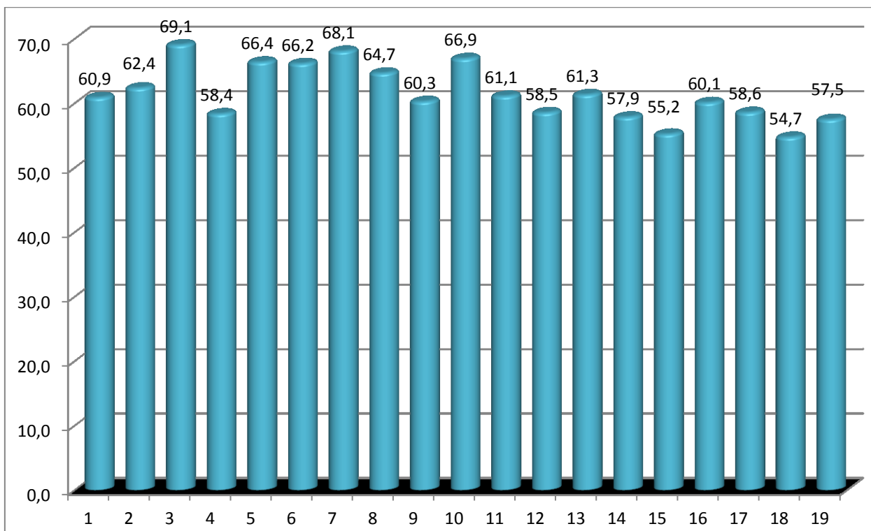
26 pav. Dienos, vakaro ir nakties triukšmo rodiklio ( L_{dvn} ) pasiskirstymas matavimo vietose. Ribinis dydis 65 dBA.
