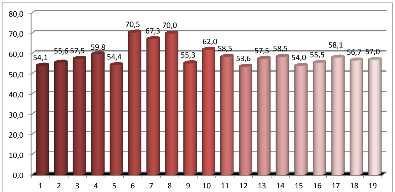
24 pav. Maksimalaus triukšmo pasiskirstymas matavimo vietose nakties metu (22-6 val.). Ribinis dydis 60 dBA.
