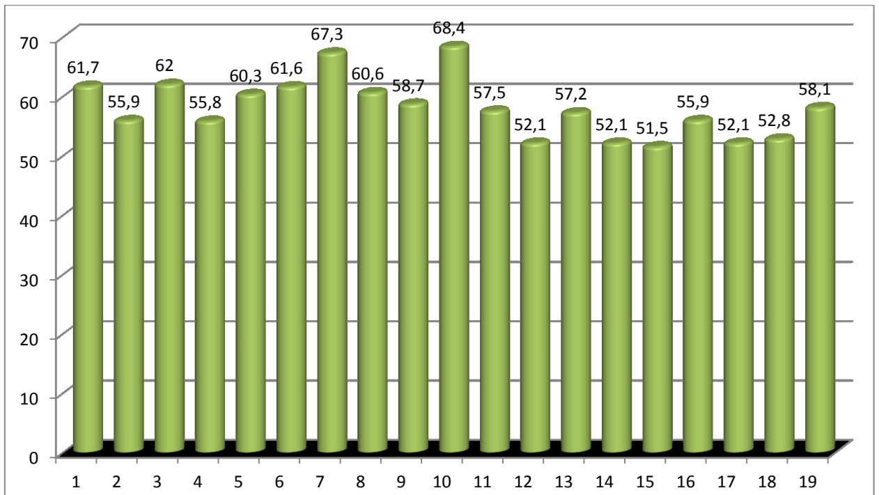
23 pav. Ekvivalentinio triukšmo pasiskirstymas matavimo vietose vakaro metu (18-22 val.). Ribinis dydis 60 dBA.
