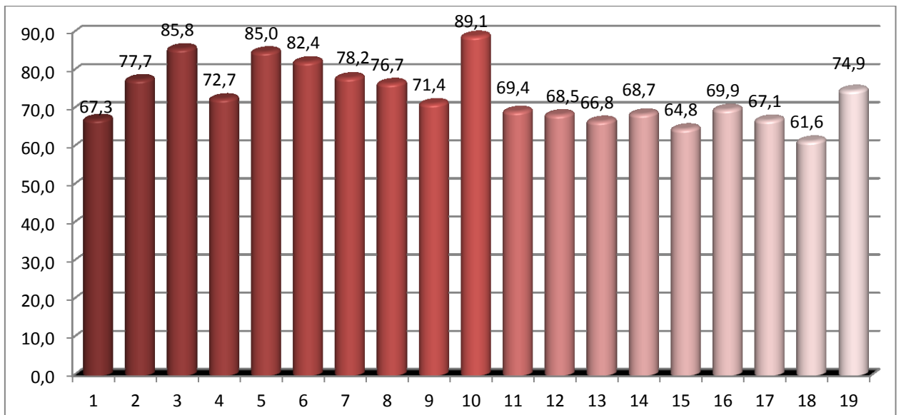
20 pav. Maksimalaus triukšmo pasiskirstymas matavimo vietose dienos metu (6-18val.). Ribinis dydis 70 dBA.
