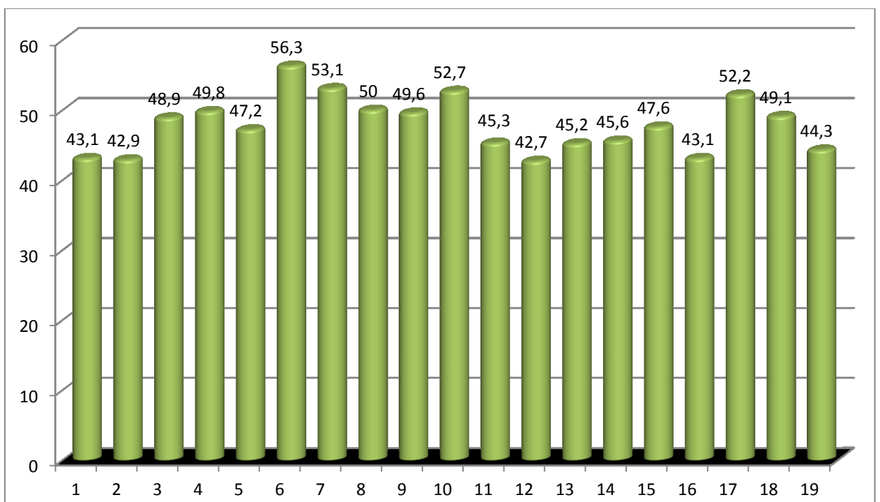
17 pav. Ekvivalentinio triukšmo pasiskirstymas matavimo vietose nakties metu (22-6 val.). Ribinis dydis 55 dBA.
