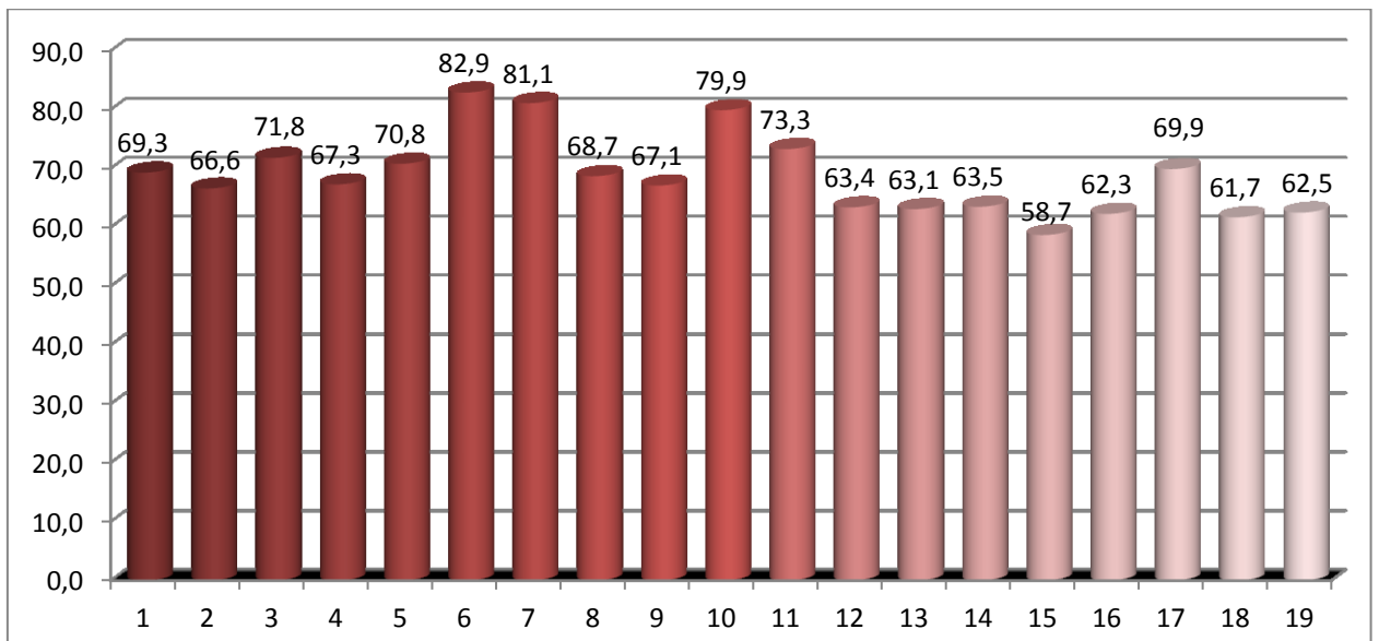
22 pav. Maksimalaus triukšmo pasiskirstymas matavimo vietose vakaro metu (18-22val.). Ribinis dydis 65 dBA.
