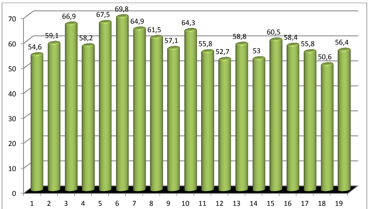
13 pav. Ekvivalentinio triukšmo pasiskirstymas matavimo vietose dienos metu (6-18 val.). Ribinis dydis 65 dBA.
