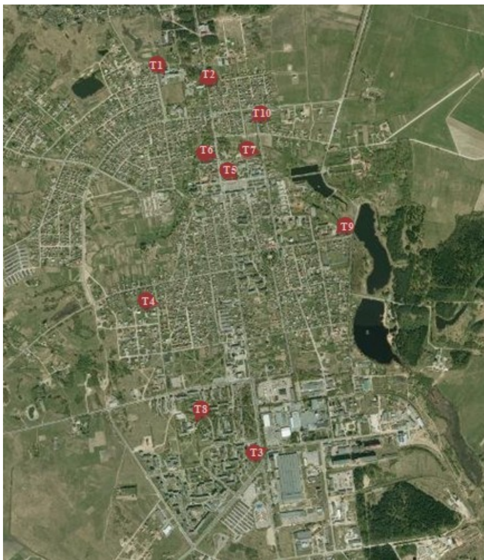
9 pav. Triukšmo matavimo vietų schema Rokiškio mieste (T1-T10)
