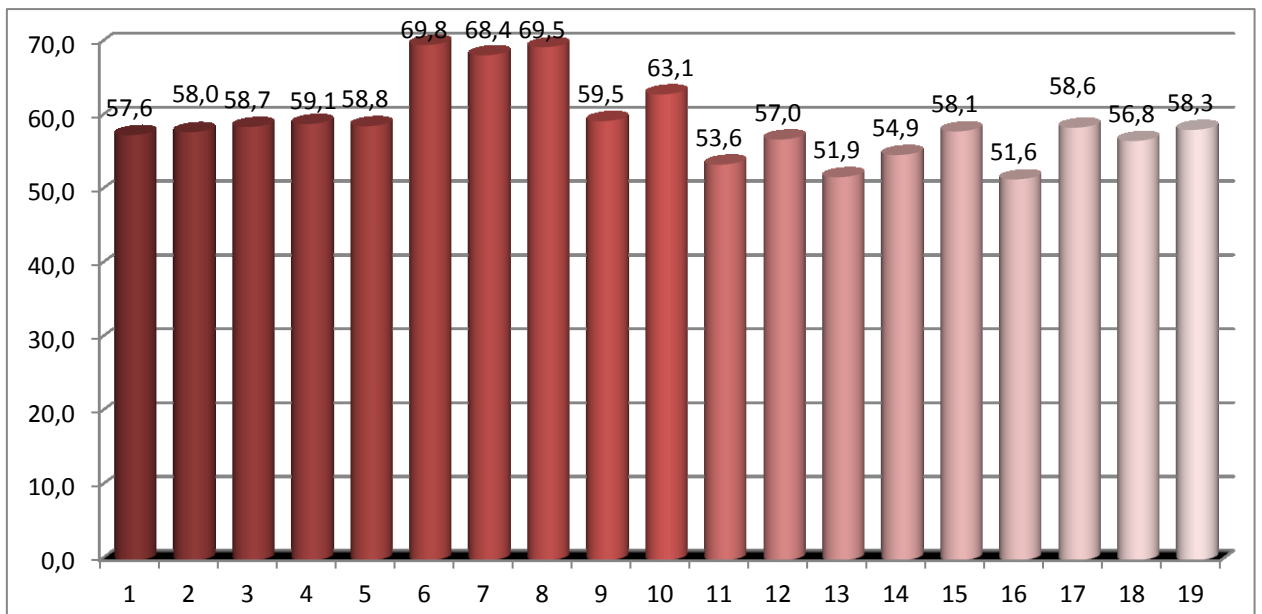
16 pav. Maksimalaus triukšmo pasiskirstymas matavimo vietose nakties metu (22-6 val.). Ribinis dydis 60 dBA.
