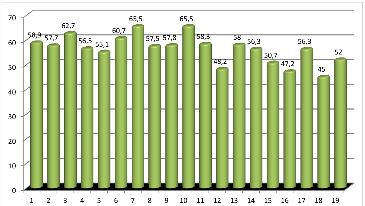
15 pav. Ekvivalentinio triukšmo pasiskirstymas matavimo vietose vakaro metu (18-22 val.). Ribinis dydis 60 dBA.
