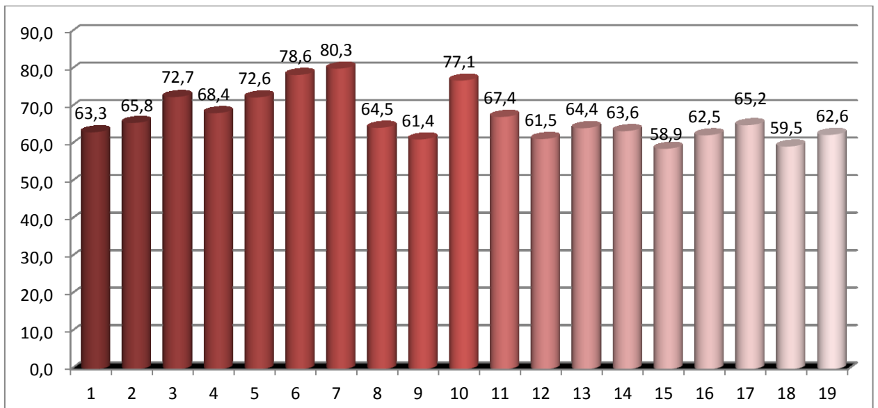
14 pav. Maksimalaus triukšmo pasiskirstymas matavimo vietose vakaro metu (18-22val.). Ribinis dydis 65 dBA.
