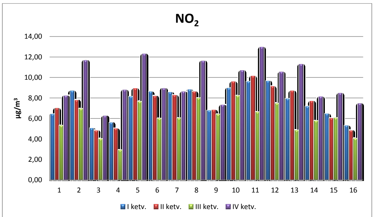
6 pav. NO 2 koncentracijų pasiskirstymai Rokiškio rajone.
